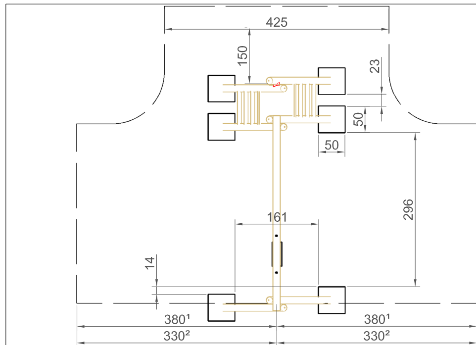
Sicherheitsbereich und Fundamentplan
