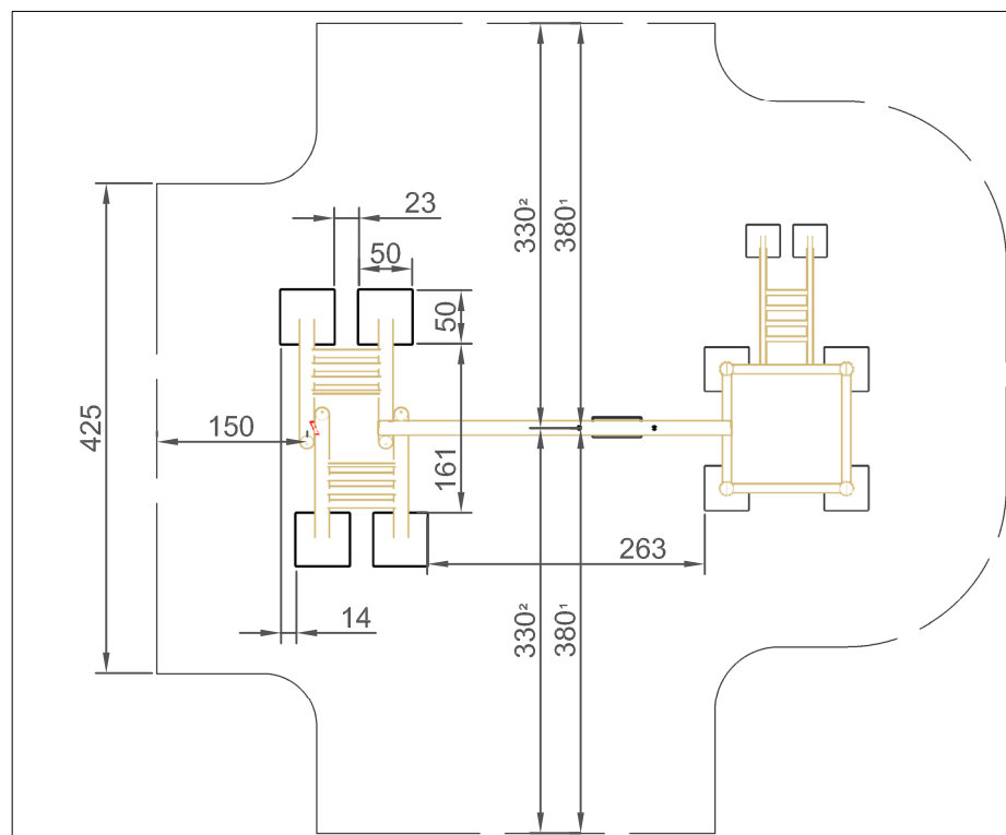
Sicherheitsbereich und Fundamentplan
